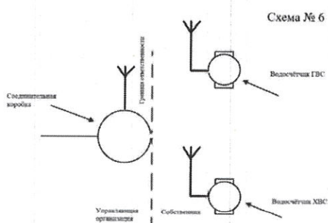
Схема № 6 Индивидуальные приборы водоучета установленные в сантехнических нишах в квартире и обслуживаются Собственником.
